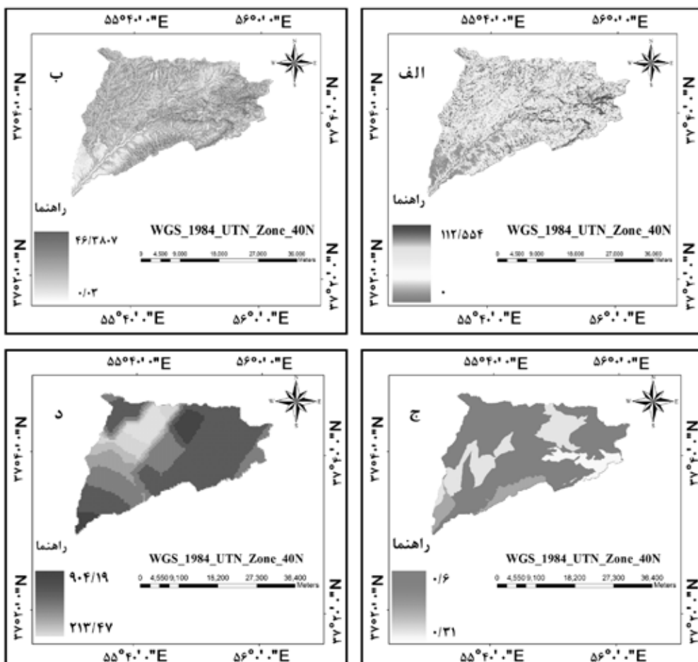
شکل ۶- نقشه‌های توانمندی فرسایش خاک بر اساس مدل فازی (الف) و مدل RUSLE (ب) و نقشه‌های خطر توانمندی فرسایش خاک بر اساس مدل فازی (ج) و مدل RUSLE (د)
