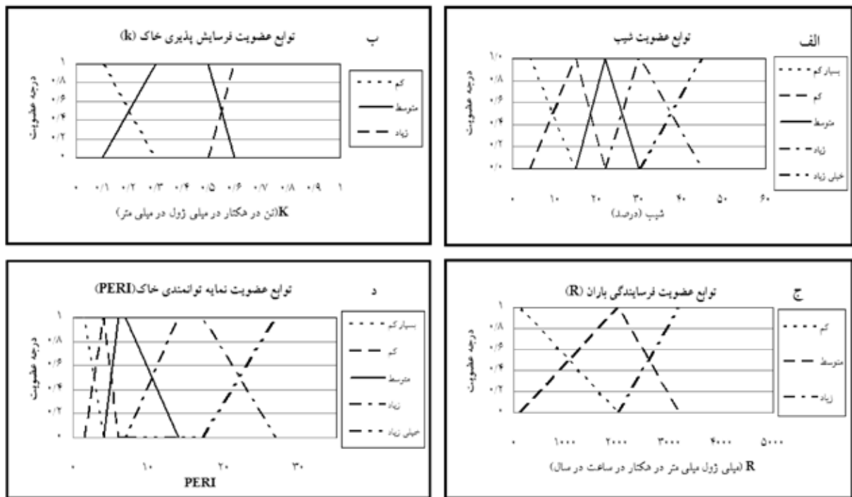
شکل ۴- توابع عضویت فازی: الف) درصد شیب، ب) فرسایش پذیری خاک، ج) فرساینندگی باران و د) نمایه توانمندی فرسایش خاک
