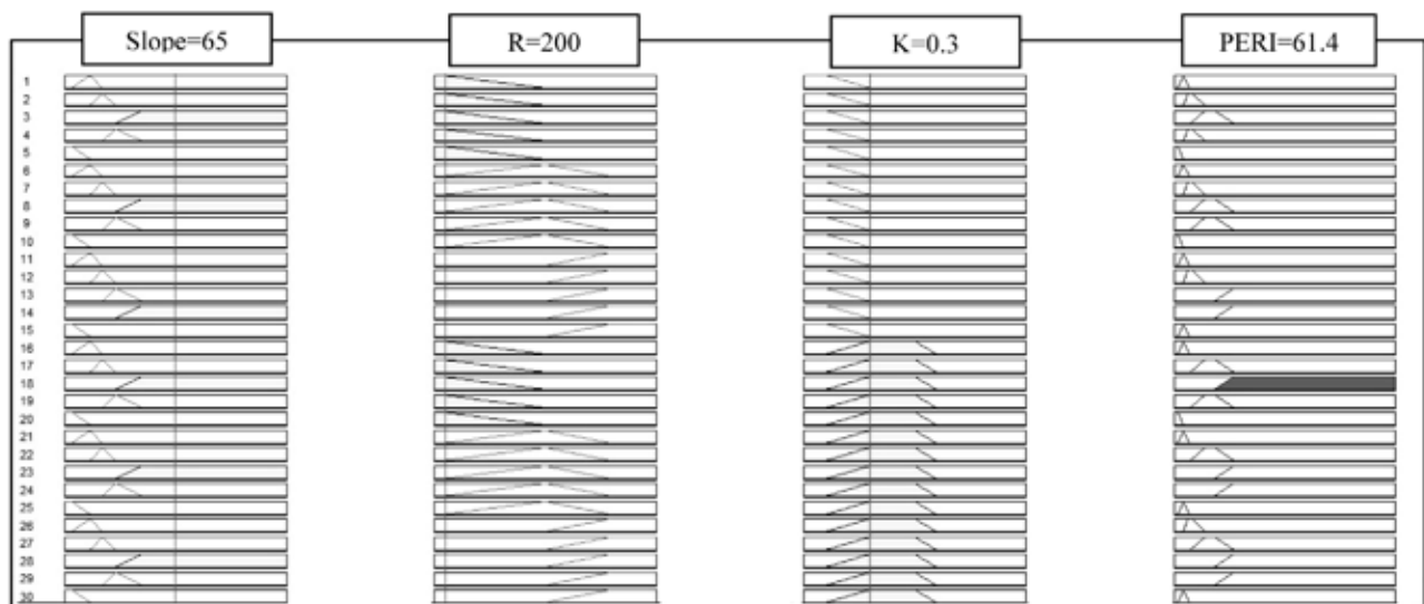
شکل ۵- محاسبه مقدار PERI برای یک پیکسل با مقادیر فرضی درصد شیب، عامل فرساینندگی باران و عامل فرسایش پذیری خاک در نرم افزار MATLAB ( فقط ۳۰ قاعده فازی در شکل نشان داده شده است)
