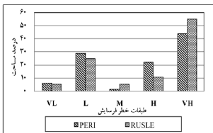
شکل ۷- مقایسه درصد طبقات مختلف خطر کل حوزه بر اساس مدل‌های فازی و RUSLE
