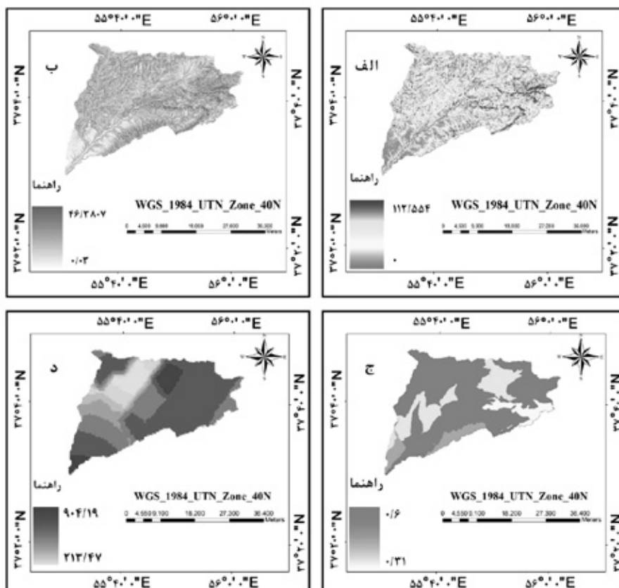
شکل ۲- عامل های ورودی: الف) درصد شیب، ب) LS، ج) فرسایش پذیری خاک (K) و د) فرساینده گی باران (R)
