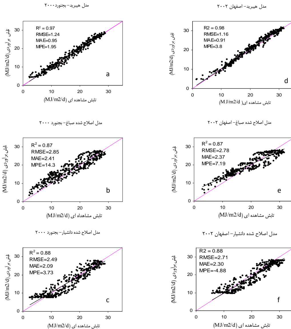
شکل ۱- مقایسه نتایج برآورد تابش روزانه خورشیدی در ایستگاههای اصفهان (۲۰۰۲) و بجنورد (۲۰۰۰) براساس مدل هبیرید و مدل‌های اصلاح شده دانشیار و صباغ در مرحله اعتبارسنجی
