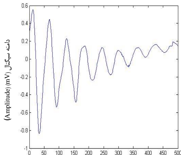
شکل ۲- سیگنال ذخیره شده در حوزه زمان
