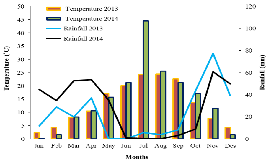
شکل ۱- میانگین بارندگی و درجه حرارت شهرستان نقده در سال ۱۳۹۲-۹۳ Fig. 1- Average rainfall and temperature of Nagadeh city in 2013-2014
