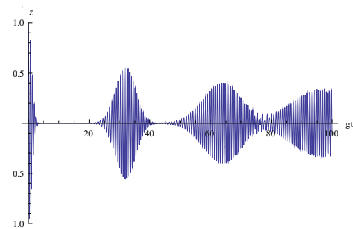
شکل ۱: تحول زمانی وارونی اتمی \langle \sigma_z \rangle برای برهم کنش اتم با میدان در حالت همدوس بر حسب زمان بهنجار شده \tau = gt و به ازای \Delta = 0 و |\alpha|^2 = 25
